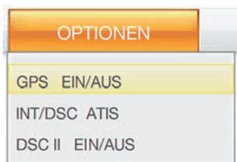
Abb. 5: IC-soft Optionsmenü
