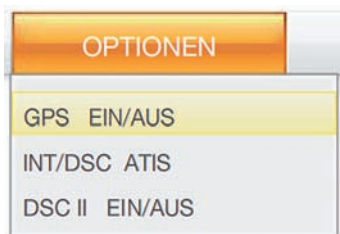
Abb. 8: IC-soft Optionsmenü
